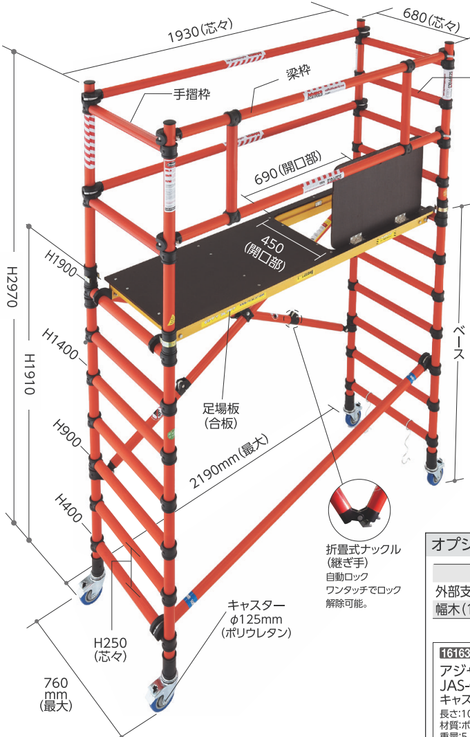
JAS-ZFG190 (1段) 単位:mm
